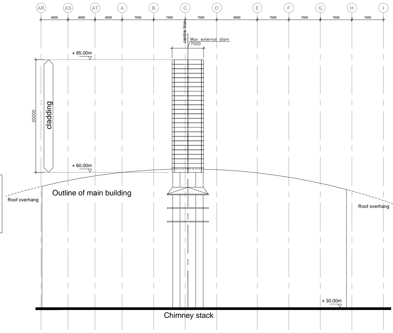
ELEVATION 1
