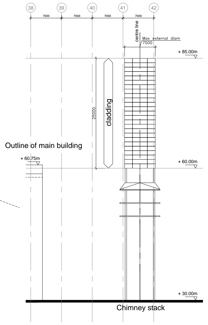
ELEVATION 2
